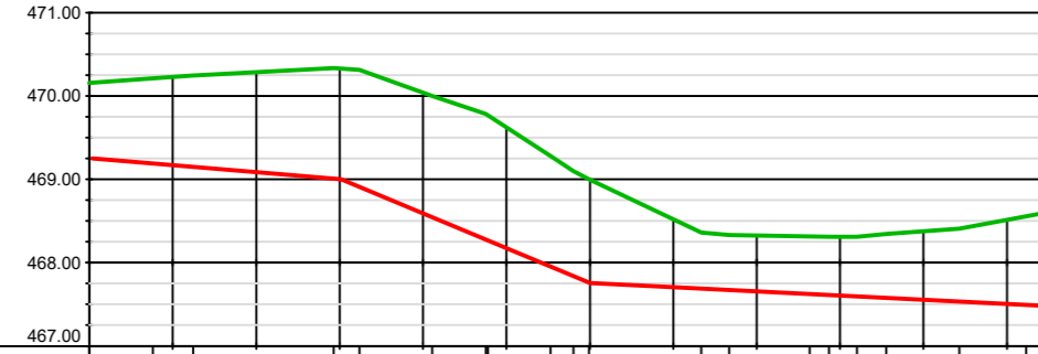
Längsschnitt Achse Graben 1 Bestand
