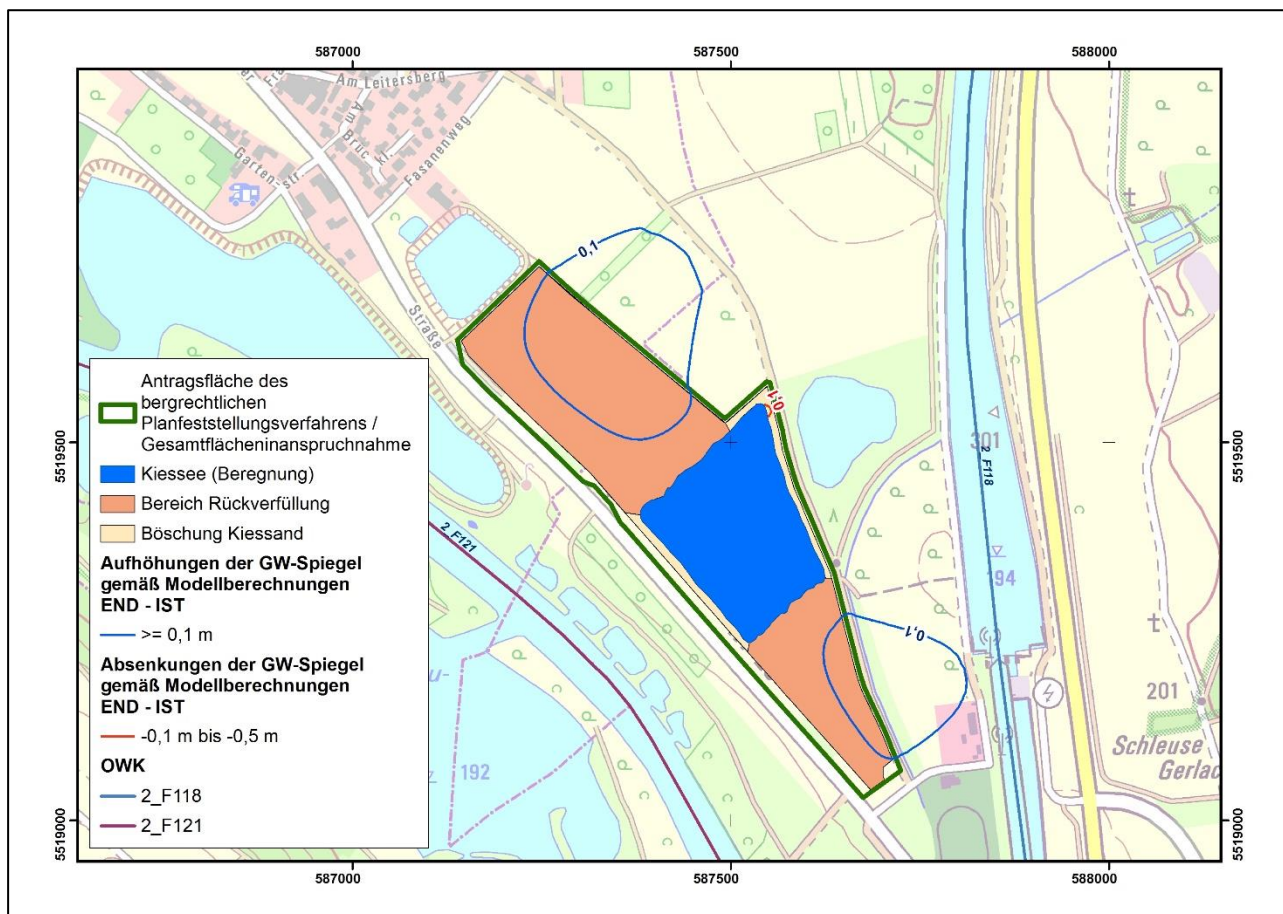
Abbildung 3-4: Modellberechnung Differenzenplan END – IST-Zustand aus /22/
