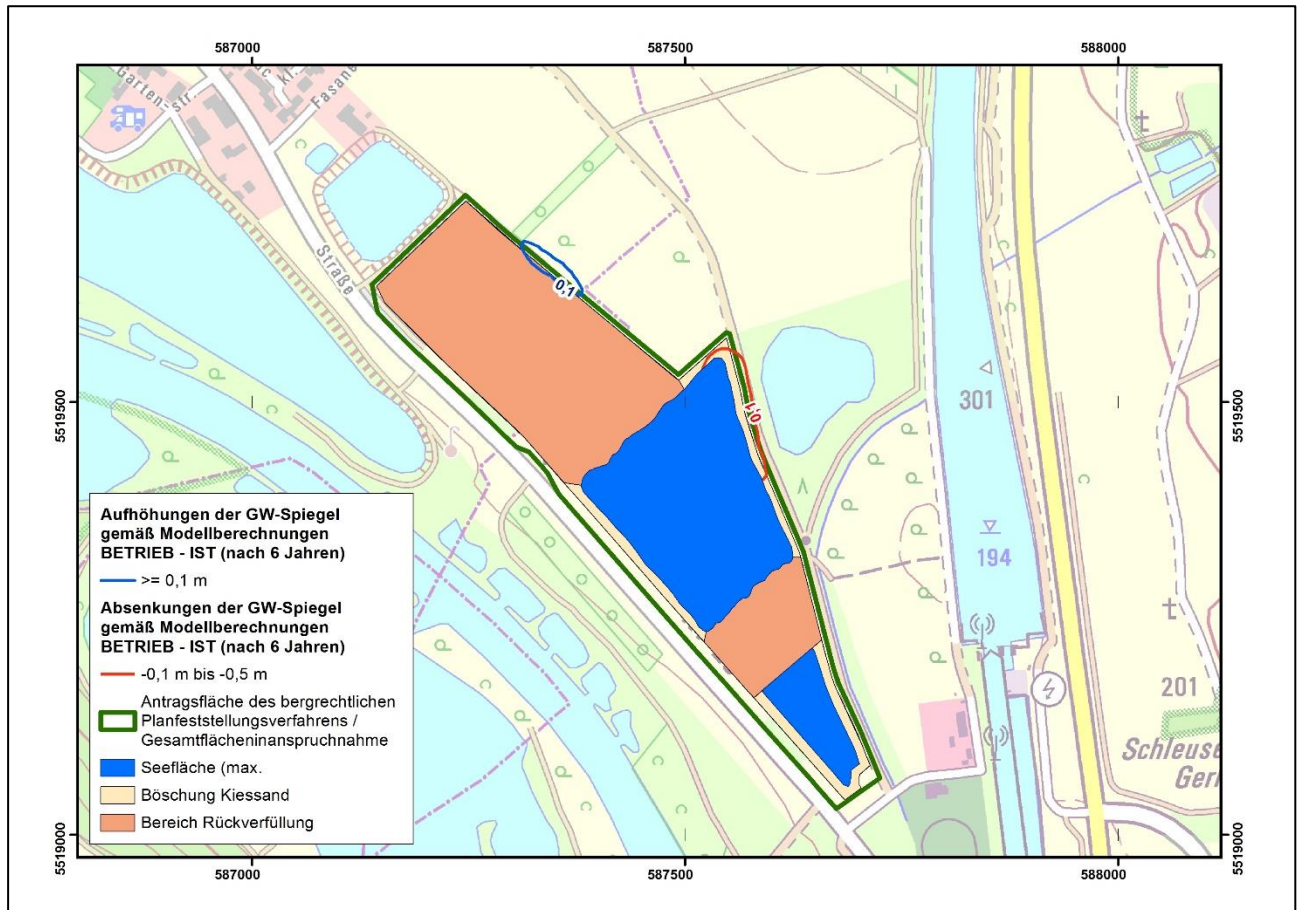
Abbildung 3-3: Modellberechnung Differenzplan BETRIEB – IST-Zustand aus /22/
